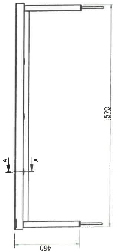
PŘEDNÍ POHLED
